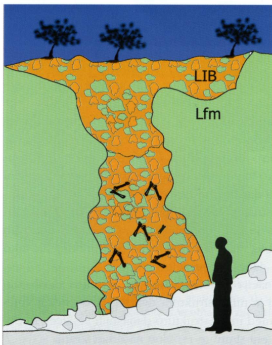
Slika 5: Skica nahajališča dinozavrov, narejena na podlagi fotografije na sliki 4. V plitvomorske apnenice Lipiške formacije (Lfm) se zajeda več kot šest metrov globok in do štiri metre širok paleokraški žep, zapolnjen z brečo, ki jo sestavljajo kosi svetlosivega apnenca Lipiške formacije, temnosivega apnenca krovne Liburnijske formacije (LIB), odlomki kosti, boksitni delci, laporasto vezivo in kalcitni cement. Fragmenti kosti se pojavljajo samo v spodnjem delu žepa. Ponekod so tako pogosti, da tvorijo kostno brečo.
