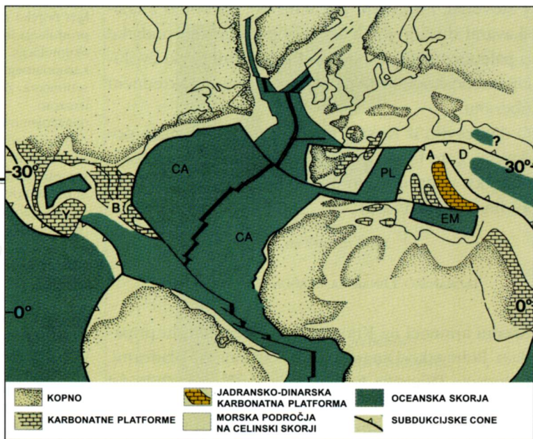
Slika 2: Paleogeografska rekonstrukcija, ki kaže položaj in razširjenost karbonatnih platform v obdobju santonija v zgornji kredi (pred 84 milijoni let). Jadransko-Dinarska karbonatna platforma je označena z rumeno. Na kontinentalnih ploščah so za orientacijo označeni obrisi današnjega kopnega. Ključ: A - Jadransko-Apulijska plošča; B - Bahami; CA - centralni Atlantik; D - Dinaridi; EM - vzhodni Mediteran; PL - Piemontsko-Ligurijski ocean; Y - Jukatan. Po Eberliju in sodelavcih (1993).
